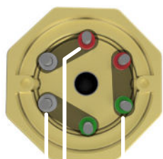
L1 L2 L3 Trekantkobling
