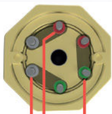
L1 L2 L3 Trekantkobling
