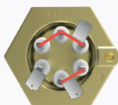
Versjon 2 2 trinn 1-fas 230V
