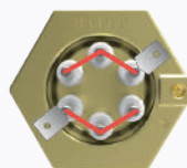
Versjon 5 1-fas 230V Skrue konektor
