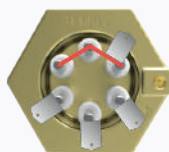
Versjon 4 Stjerne 3-fas 400V
