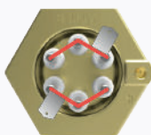
Versjon 3 1 fas 230 V
