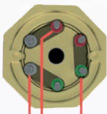
L1 L2 L3 Trekantkobling
