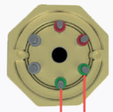
L1 L2 1-fase element
