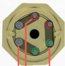
L1 L2 L3 Trekantkobling
