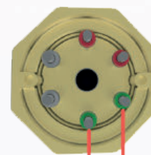
L1 L2 1-fase element
