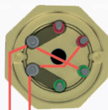
L1 L2 1-fase 3 elementer
