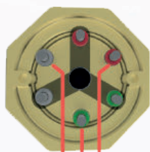
L1 L2 L3 Stjernekobling
